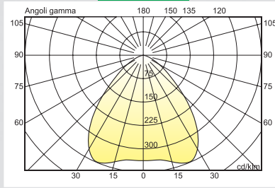
VOGUE VD 150W MT
