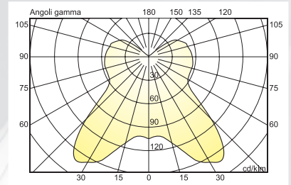
VOGUE GTA-TI/40 150W ME
