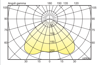
VOGUE RP 57W FSM
